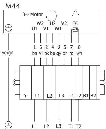
Fig.: Triphasé, enroulement pour 2 tensions, montage triangle
