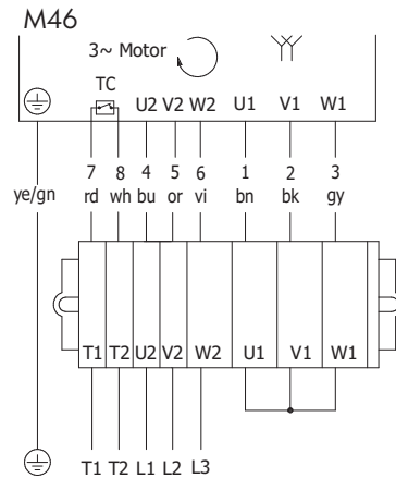
Fig.: Triphasé, câble 7+2 conducteurs, 2 vitesses, montage double étoile
