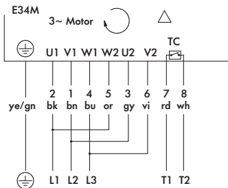
Fig.: Triphasé, câble 7+2 conducteurs, enroulement pour 2 tensions, montage triangle
