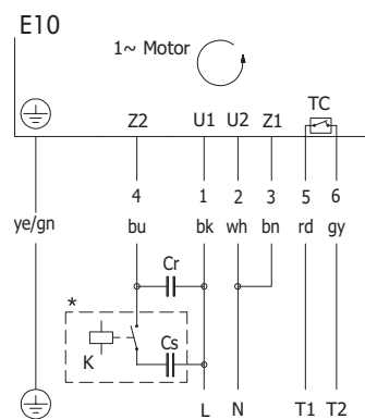
Fig.: Monophasé, câble 7 conducteurs
