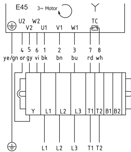
Fig.: Triphasé, câble 9 conducteurs, enroulement pour 2 tensions, montage étoile
