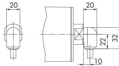
Fig.: Presse-étoupe coudé, technopolymère
