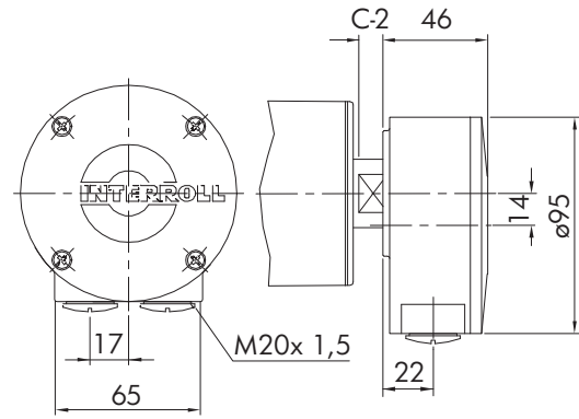
Fig.: Boîte à bornes, aluminium
