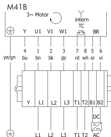
Fig.: Avec frein, triphasé, enroulement pour 1 tension, montage étoile
