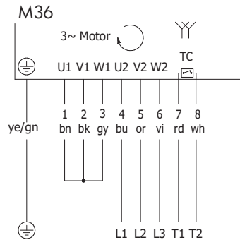
Fig.: Triphasé, câble 7+2 conducteurs, 2 vitesses, montage double étoile
