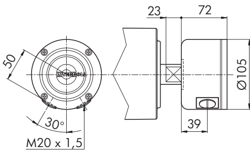
Fig.: Boîte à bornes, technopolymère
