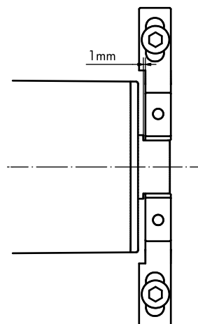
Fig.: Jeu axial maximal
