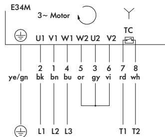
Fig.: Triphasé, câble 7+2 conducteurs, enroulement pour 2 tensions, montage étoile
