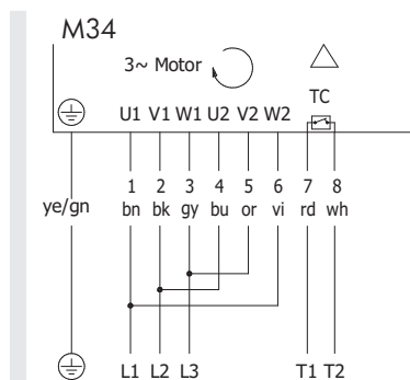
Fig.: Triphasé, câble 7+2 conducteurs, enroulement pour 2 tension, montage triangle
