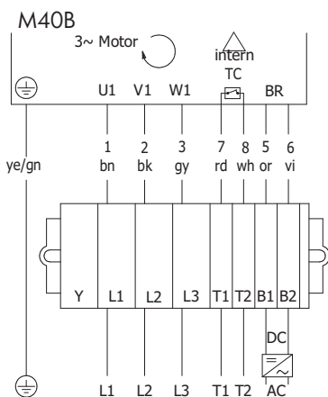
Fig.: Avec frein, triphasé, enroulement pour 1 tension, montage triangle
