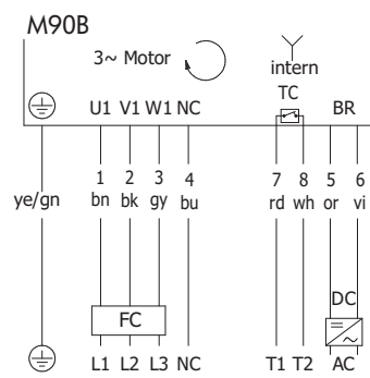
Fig.: Triphasé, câble 7+2 conducteurs, enroulement pour 1 tension, montage étoile
