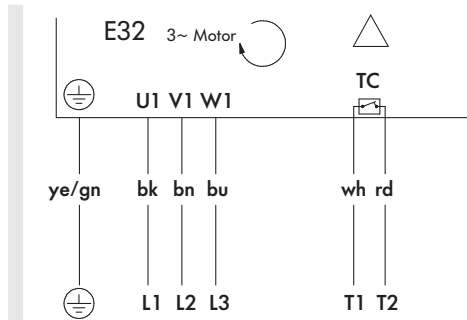
Fig.: Triphasé, câble 6 conducteurs, enroulement pour 1 tension, montage triangle
