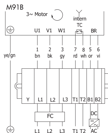
Fig.: Avec frein, triphasé, câble 7+2 conducteurs, enroulement pour 1 tension, montage étoile
