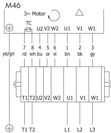
Fig.: Triphasé, câble 7+2 conducteurs, 2 vitesses, montage triangle
