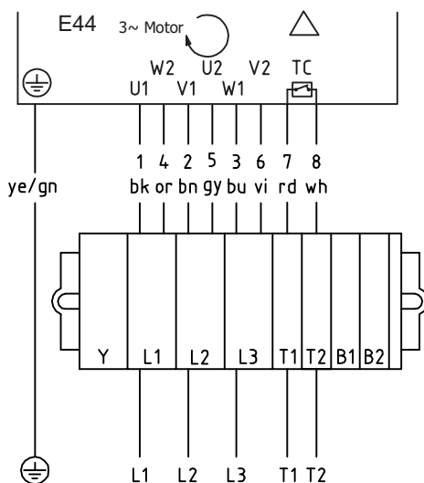
Fig.: Triphasé, câble 9 conducteurs, enroulement pour 2 tensions, montage triangle
