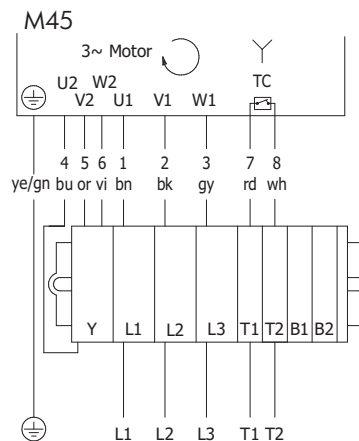
Fig.: Triphasé, enroulement pour 2 tensions, montage étoile
