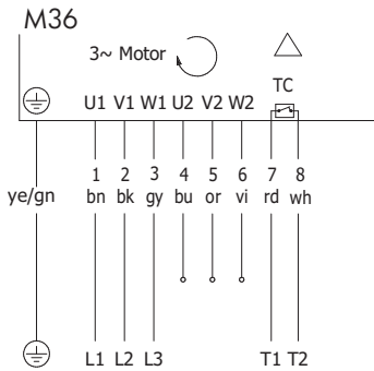
Fig.: Triphasé, câble 7+2 conducteurs, 2 vitesses, montage triangle
