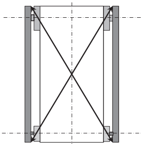
Fig.: Contrôle dans le sens diagonal
