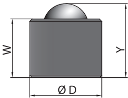
齐平安装（压合）
