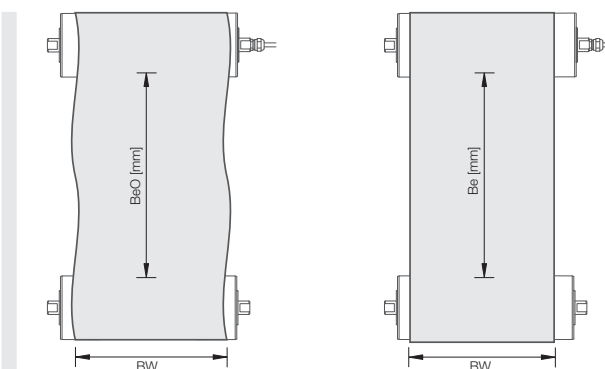
图：测量皮带伸长度
