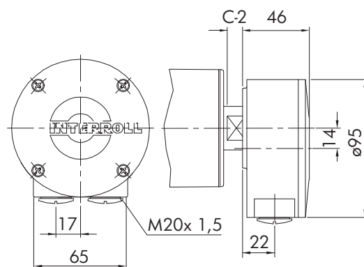
图：接线盒，铝
