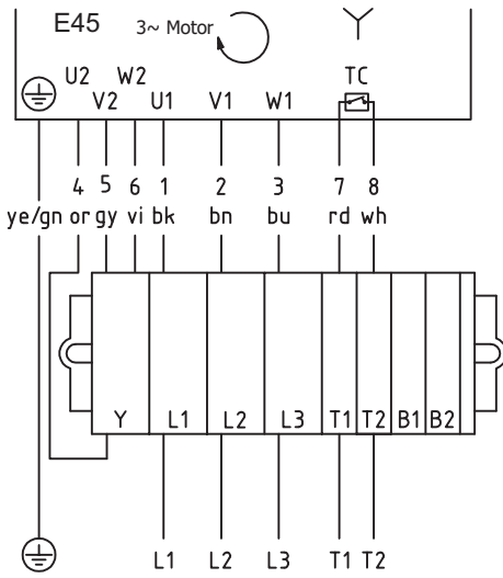
图：3 相，9 芯电缆，双电压绕组，星形连接
