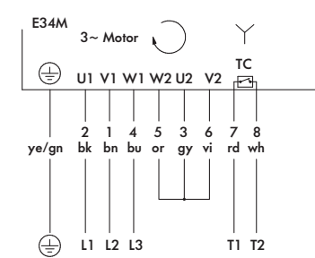
图：3 相，7+2 芯电缆，双电压绕组，星形连接
