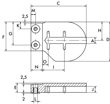
图：左侧支架 (B) PE
