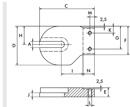
尺寸 DM 0080
