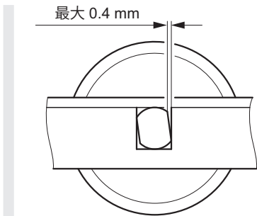
图：最大扭转间隙
