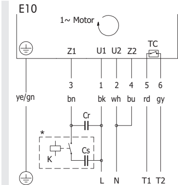
图：1 相，7 芯电缆
