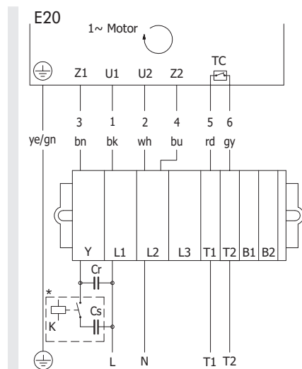
图：1 相，7 芯电缆
