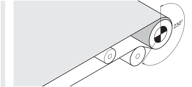
图：摩擦驱动皮带输送机增大后的皮带包角
