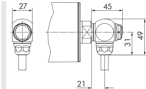
图：90° 卫生连接器，IP69k 不锈钢
