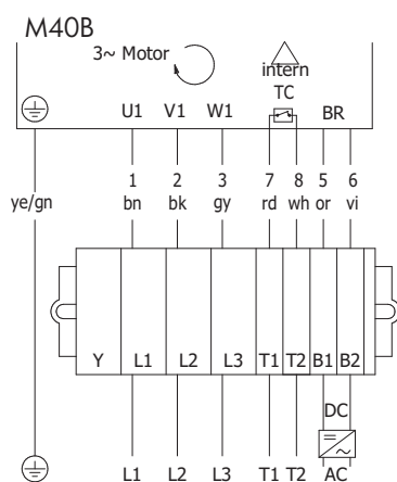
图：带制动，3 相，单电压绕组，三角形接法
