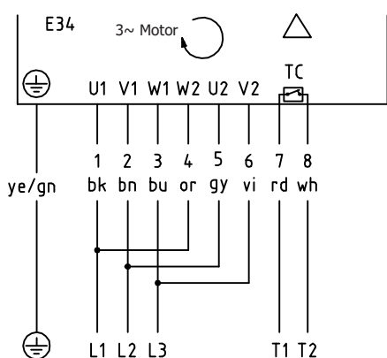
图：3 相，9 芯电缆，双电压绕组，三角形连接
