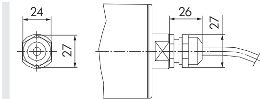
图：直管接头，黄铜或不锈钢
