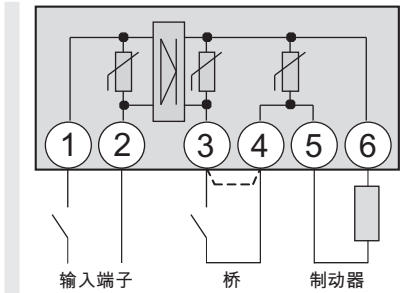
图：桥式整流器
