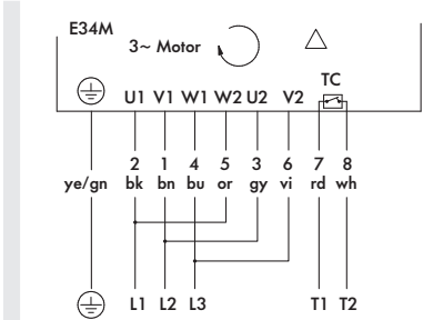
图：3 相，7+2 芯电缆，双电压绕组，三角形连接
