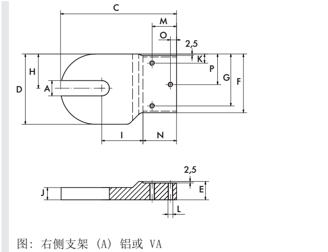
DM 0113、DM 0138 和 DM 0165 尺寸
