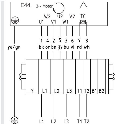
图：3 相，9 芯电缆，双电压绕组，三角形连接
