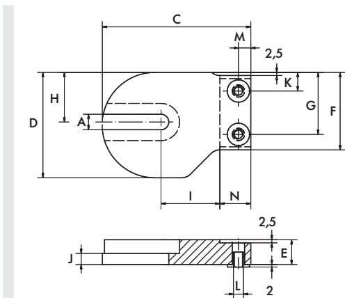
图：右侧的支架（A）PE
