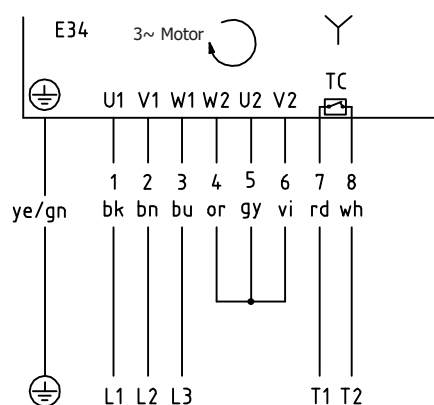
图：3 相，9 芯电缆，双电压绕组，星形连接
