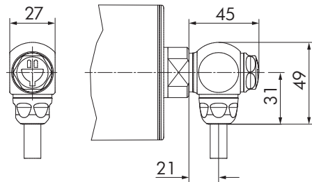
图：90° 插接头连接，符合卫生清洁标准，IP69k 不锈钢
