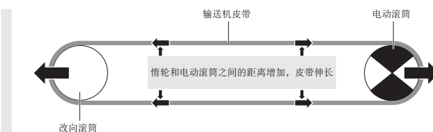
图：皮带伸长度
