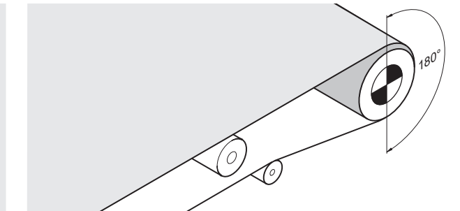
图：摩擦驱动皮带输送机的最小皮带包角
