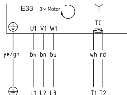
图：3 相，6 芯电缆，单电压绕组，星形连接
