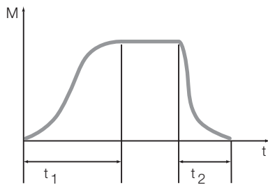
图：关闭和打开响应时间
