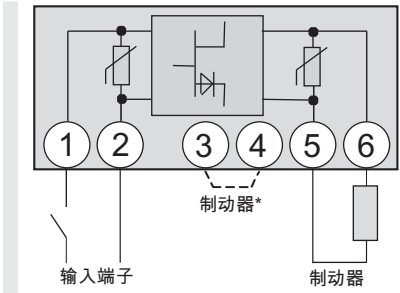
图：相位整流器
