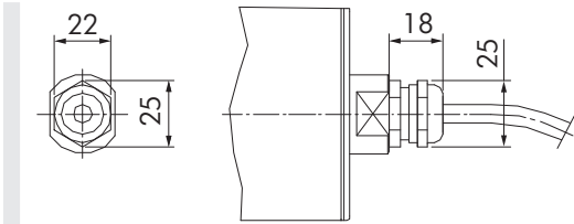
图：直型 EMC 接头，黄铜或不锈钢
