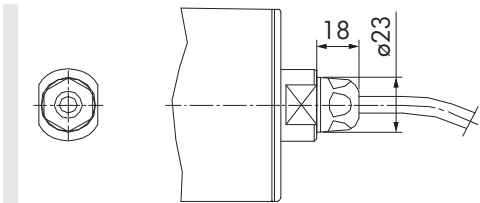
图：直管卫生接头，IP69k 不锈钢
