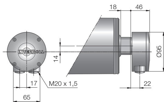
图：接线盒，铝
