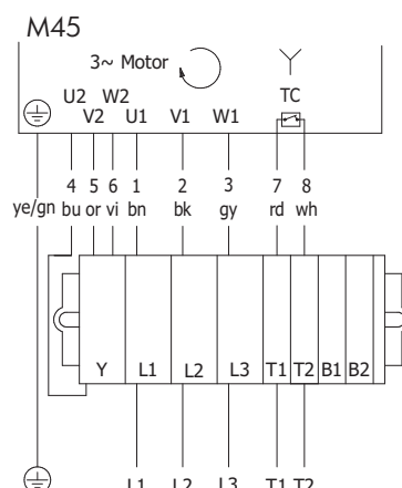
图：3 相，双电压绕组，星形接法
