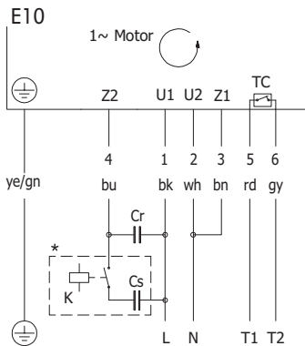
图：1 相，7 芯电缆
