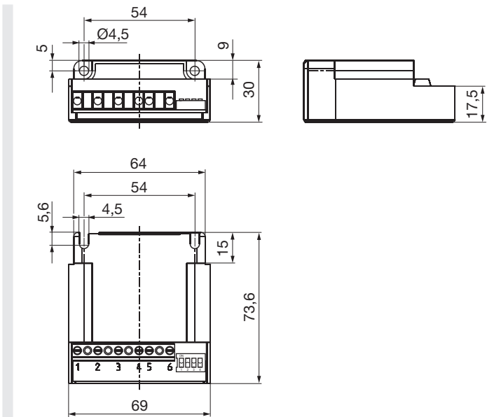
多路开关整流器
