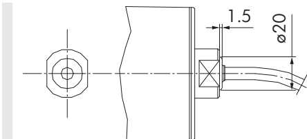
图：直型 EMC 接头，黄铜或不锈钢
