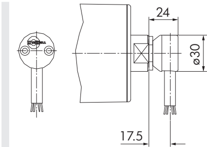
图：肘形连接器，不锈钢，也用于编码器
