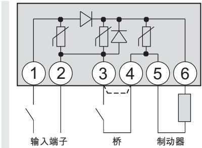
图：半波整流器
