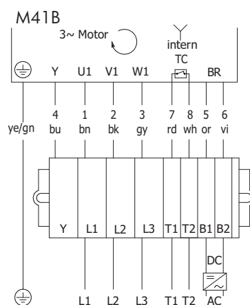
图：带制动，3 相，单电压绕组，星形接法
