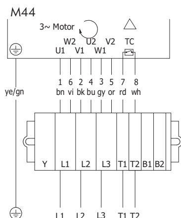
图：3 相，双电压绕组，三角形接法
