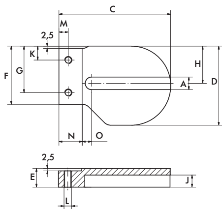
图：左侧支架 (B) 铝或 VA
