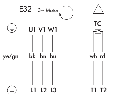
图：3 相，6 芯电缆，单电压绕组，三角形连接
