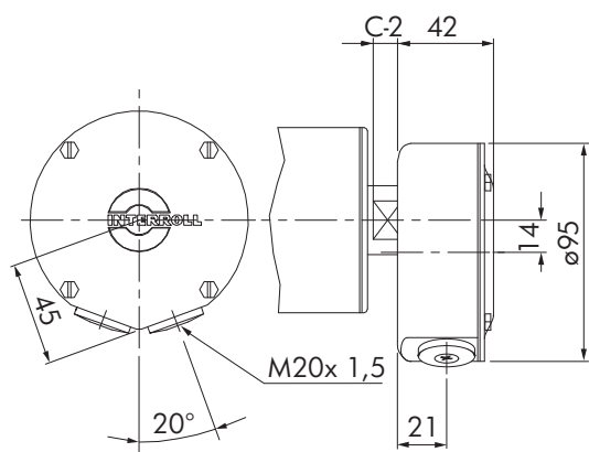
图：接线盒，不锈钢
