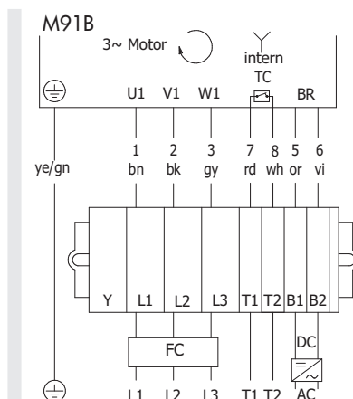
图：带制动，3 相，7+2 芯电缆，单电压绕组，星形接法
