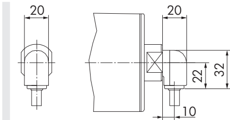
图：弯管接头，高分子聚合物
