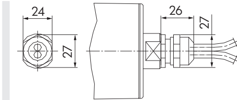
图：编码器的直管接头，黄铜或不锈钢
