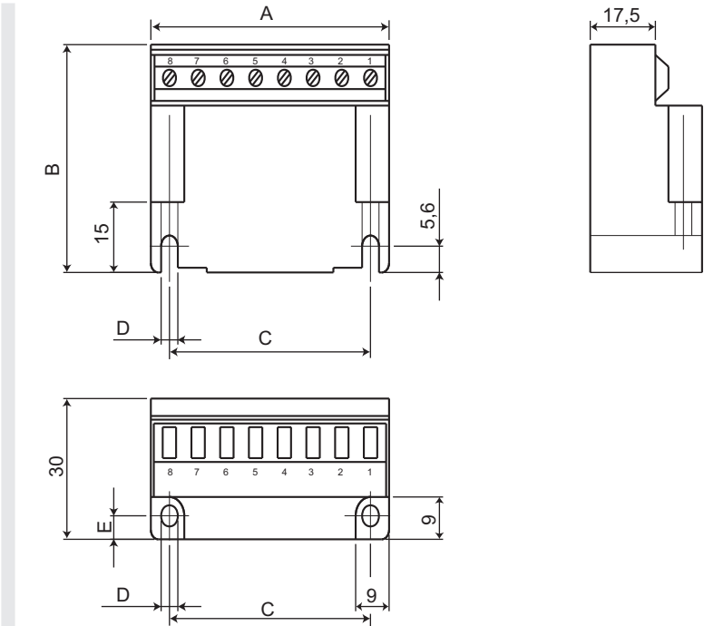
快速整流器
