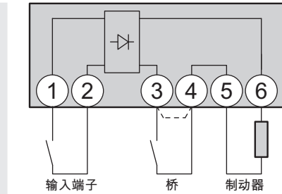
图：多路开关整流器
