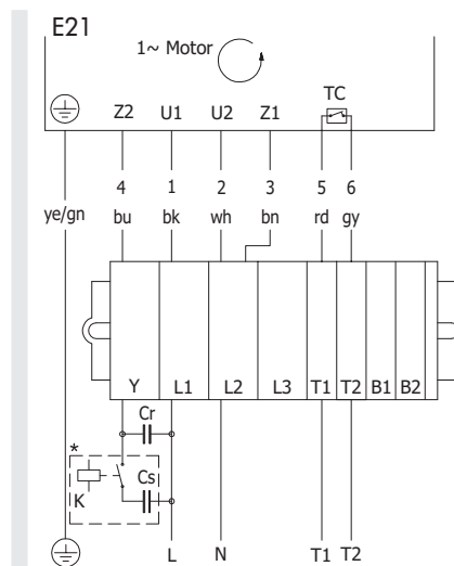
图：1 相，7 芯电缆
